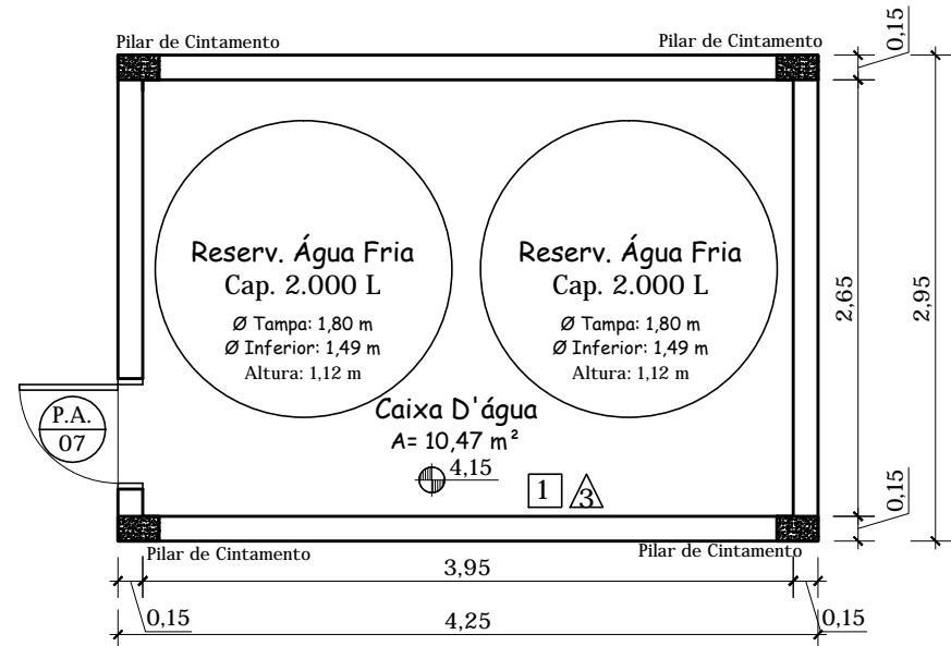
Planta Baixa das Caixas D'água Área: 12,54 m²
