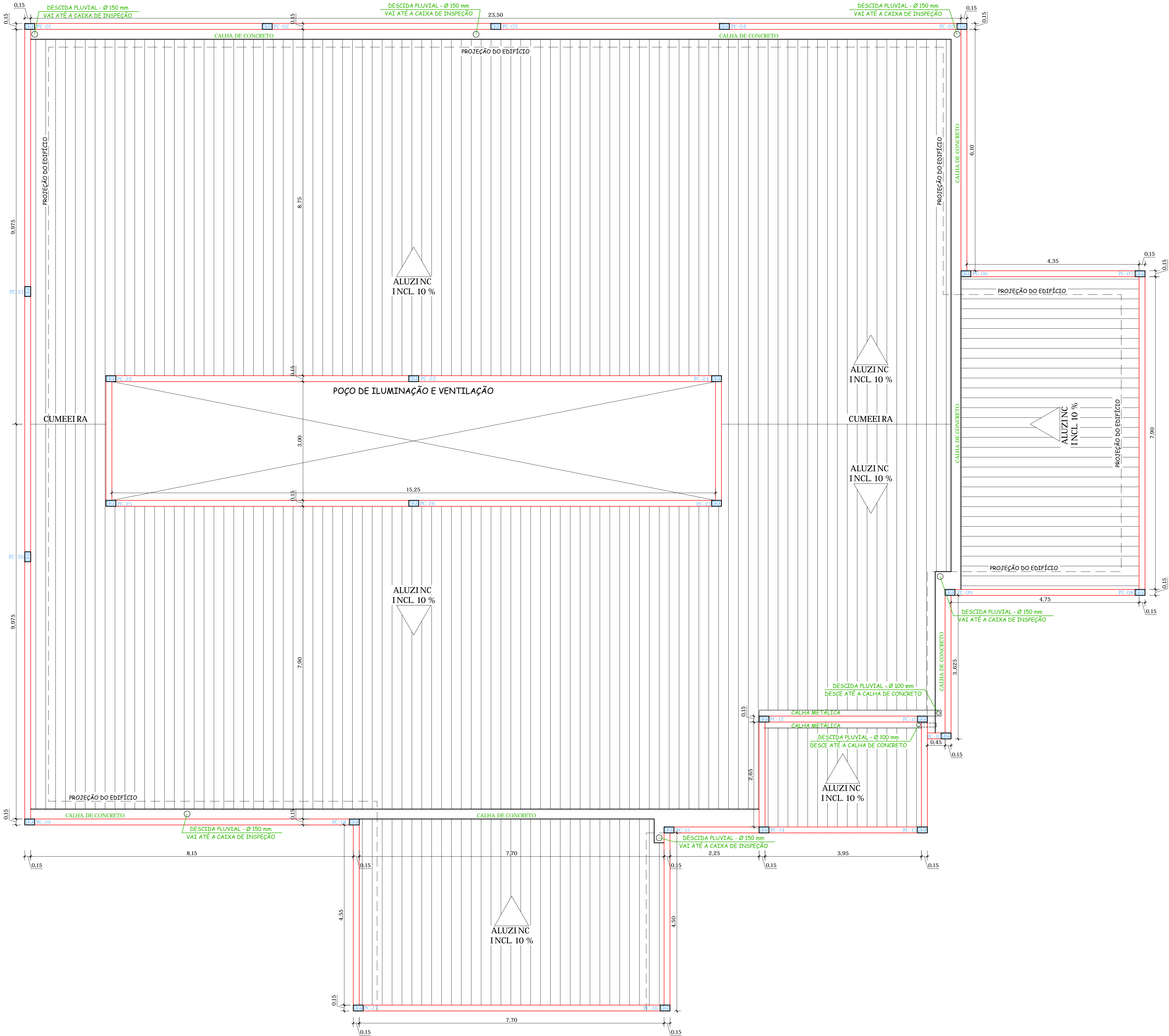
Planta de Cobertura
